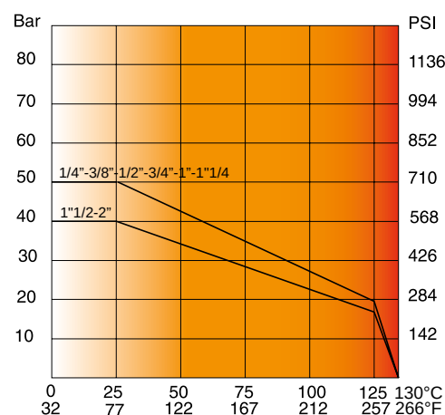
Diagramma pressione/temperatura
