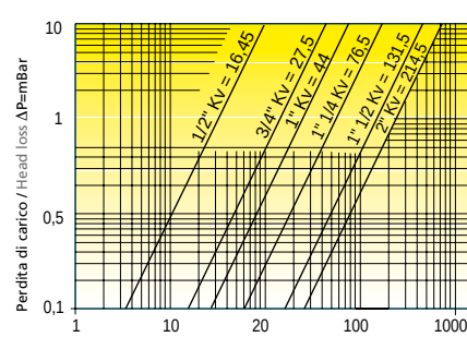
Diagramma perdite di carico (prova eseguita con aria) Head loss diagram (tested with air)
